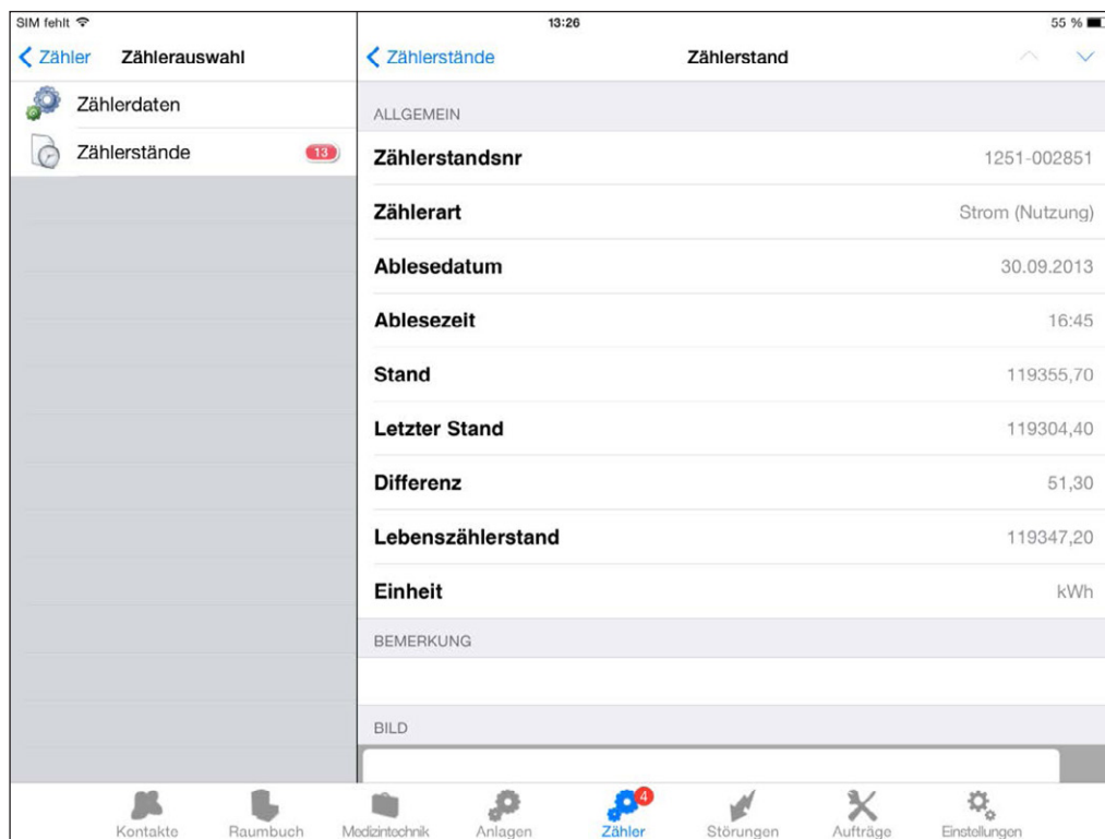
Abbildung 32 / Zählerstand Detailsicht
